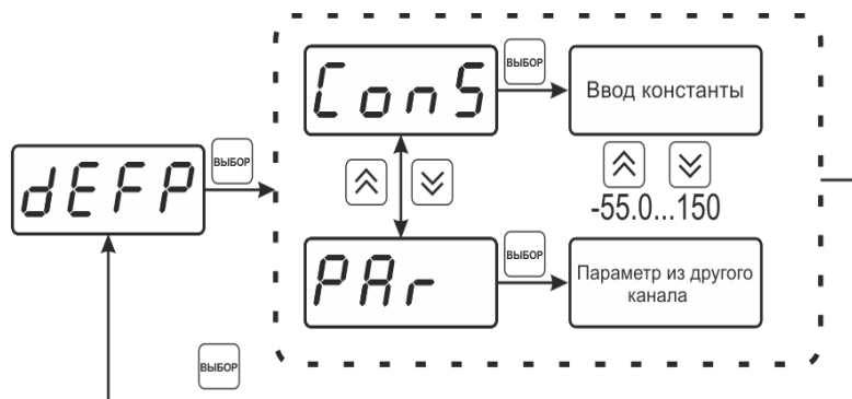
Рисунок 6.33 Введение постоянного параметра регулирования
