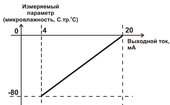
Рисунок 6.31 Пример настройки линейного выхода
