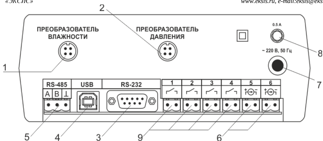
Рисунок 3.2 Задняя панель прибора (ИБГ-1 /1-C-2А, ИБГ-1 /1-C-4Р-2А (сверху вниз)
