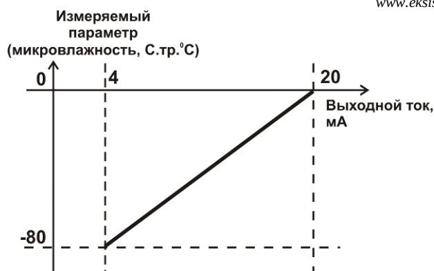
Рисунок 3.15 Линейный выход 4...20 мА по диапазону влажности -80...0 °С по точке росы
