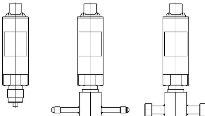
Рисунок 3.18 Измерительные преобразователи давления ИПД-02, ИПД-02-М8, ИПД-02-М16 (по порядку слева направо)
