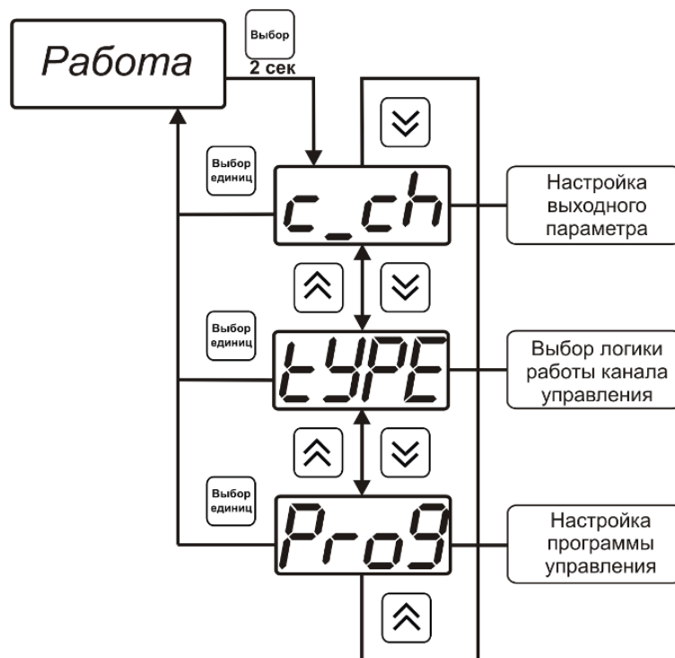
Рисунок 6.23 Режим настройки канала регулирования
