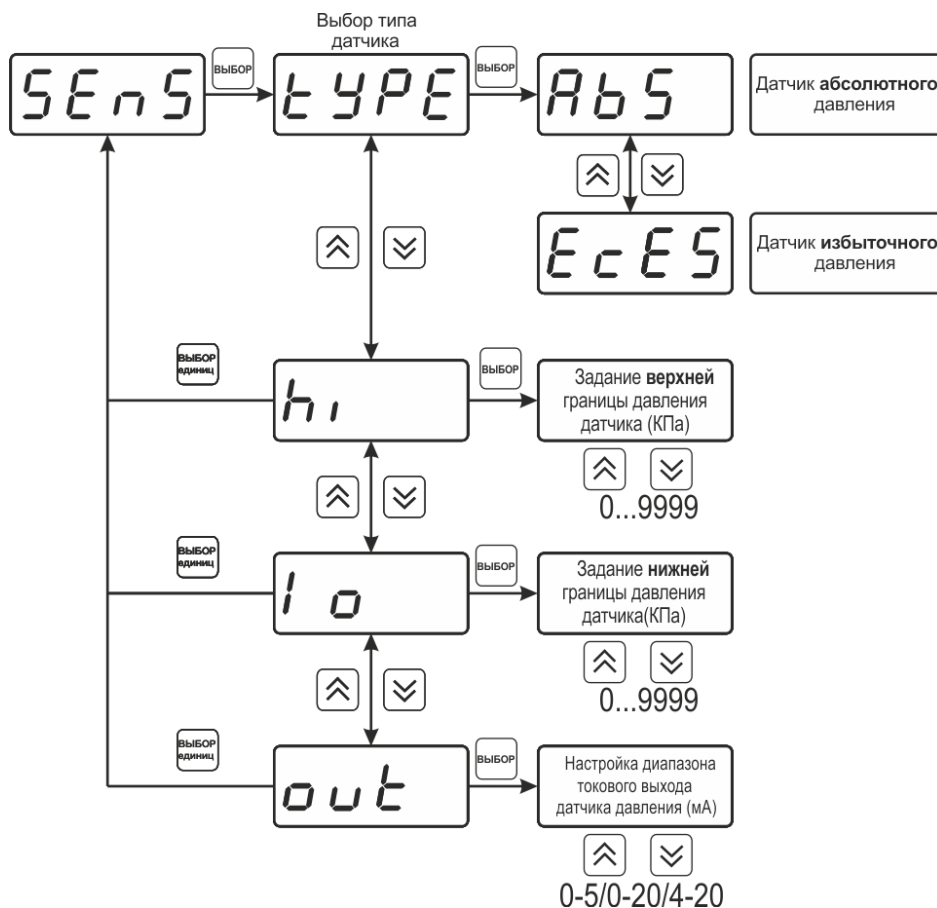
Рисунок 6.14 - Настройки параметров датчика давления
