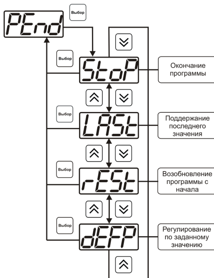
Рисунок 6.37 Меню настройки условий окончания программы
