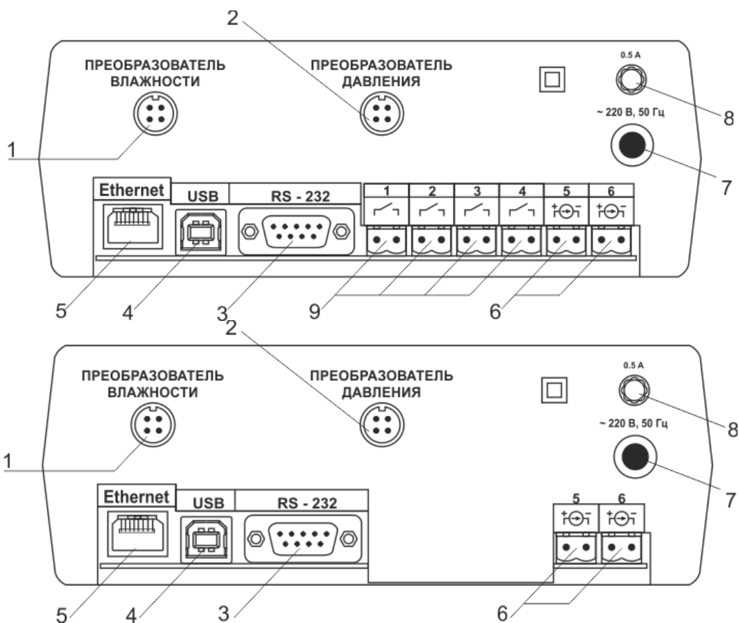
Рисунок 3.3 Задняя панель прибора (ИБГ-1 /1-C-2А, ИБГ-1 /1-C-4Р-2А (сверху вниз)
