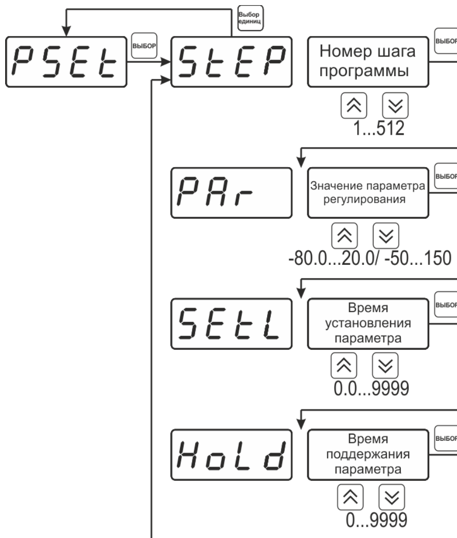
Рисунок 6.39 Меню настройки программы
