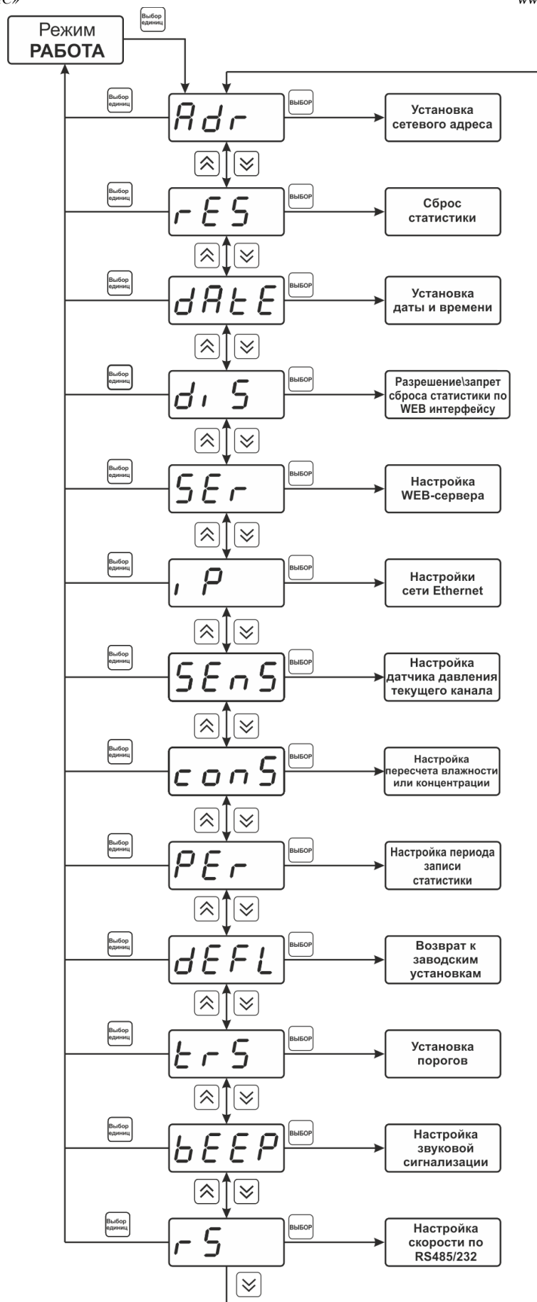
Рисунок 6.5 Режим настройки общих параметров прибора
