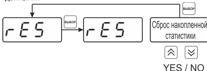
Рисунок 6.7 Меню сброса статистики
