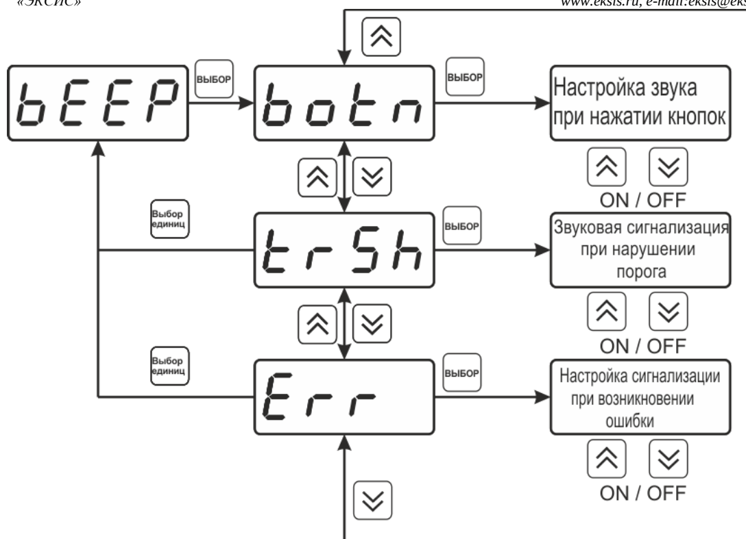
Рисунок 6.21 Настройки звуковой сигнализации
