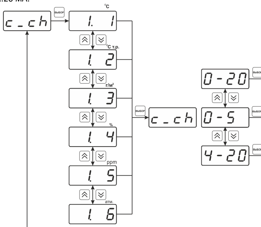
Рисунок 6.25 Настройка входного параметра канала управления (токовый)
