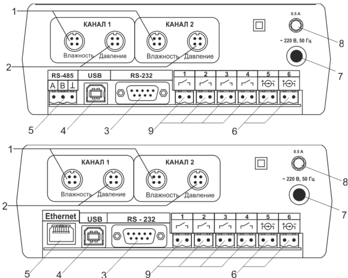
Рисунок 3.4 Задняя панель приборов ИВГ-1 /1-С, ИВГ-1 /2-С.
