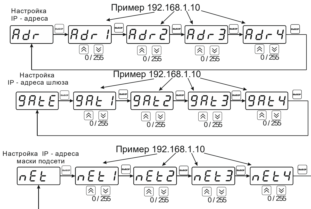
Рисунок 6.12 Меню сетевых настроек
