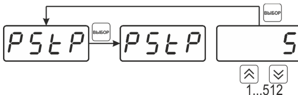
Рисунок 6.36 Задание последнего шага программы
