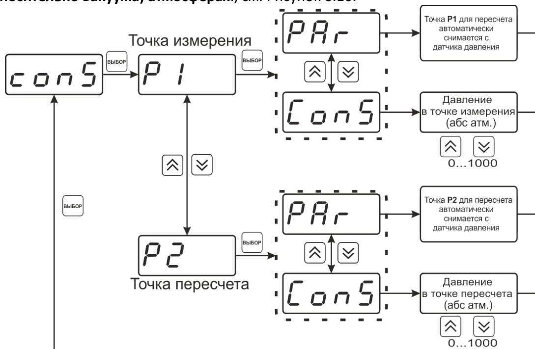
Рисунок 6.16 - Настройка пересчета влажности
