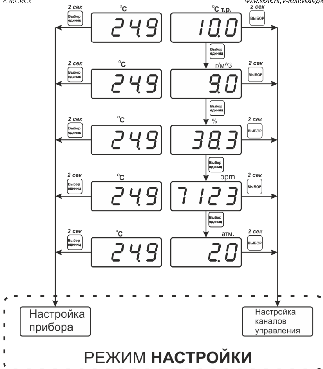
Рисунок 6.1 Режим РАБОТА для одноканального исполнения
