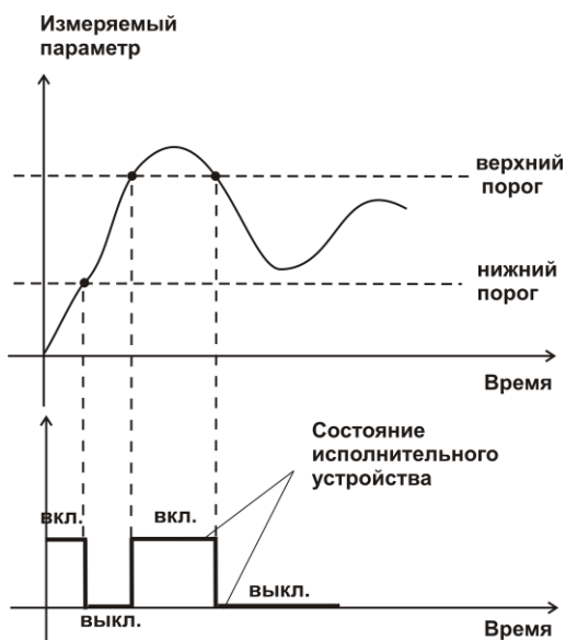
Рисунок 3.13 Функция вида f = НП + ВП
