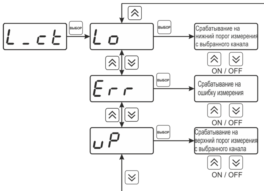
Рисунок 6.28 Настройка логического сигнализатора
