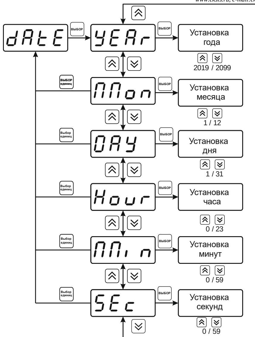
Рисунок 6.8 Настройка даты и времени
