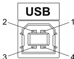
Рисунок 3.7 Разъем USB (розетка «В»)
