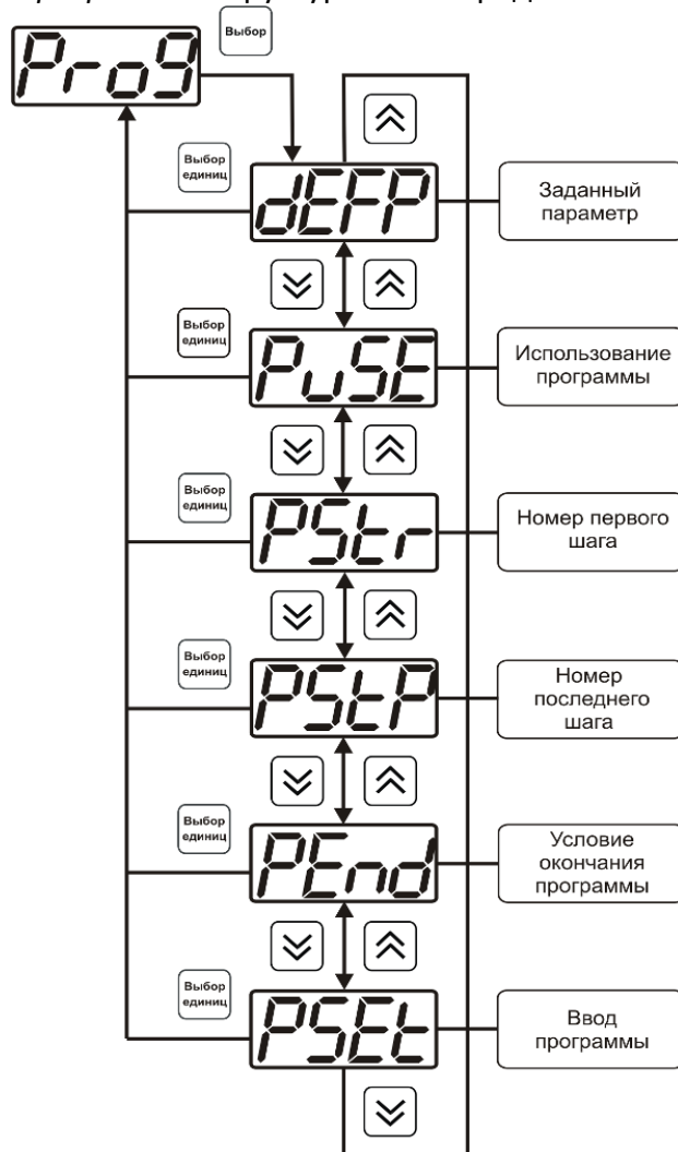
Рисунок 6.32 Меню настройки программы управления
