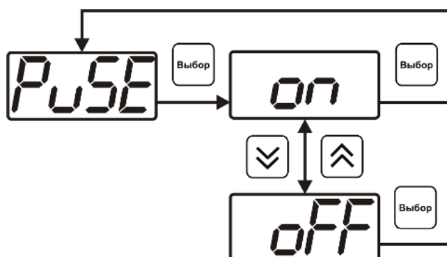
Рисунок 6.34 Включение/выключение регулирования по программе
