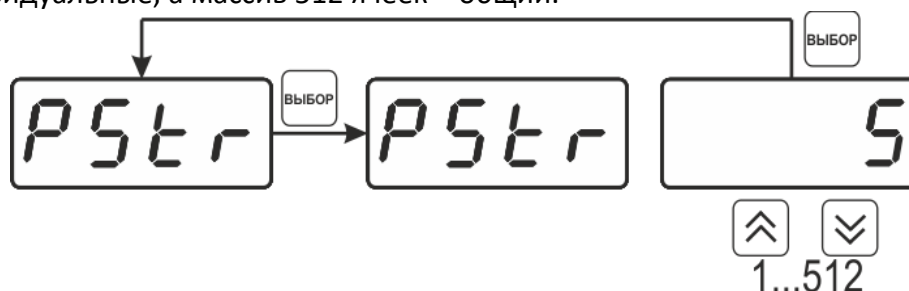
Рисунок 6.35 Задание стартового шага программы
