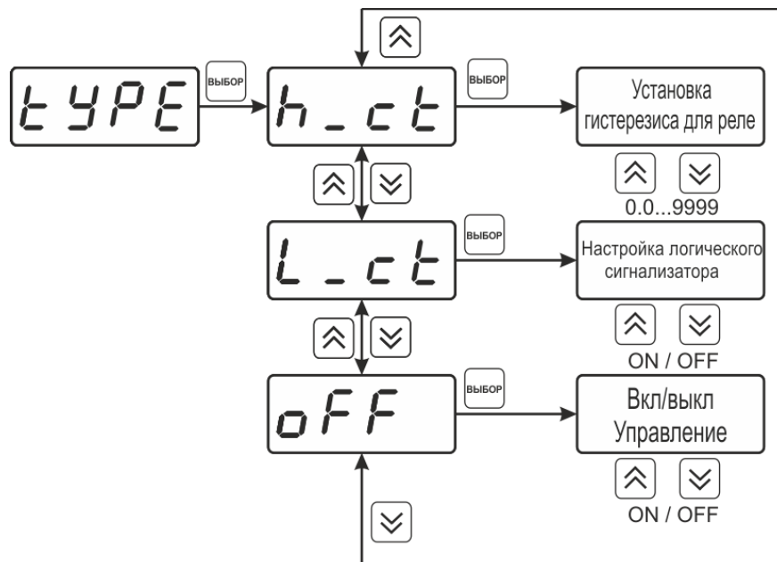
Рисунок 6.26 Выбор логики работы канала управления (реле)
