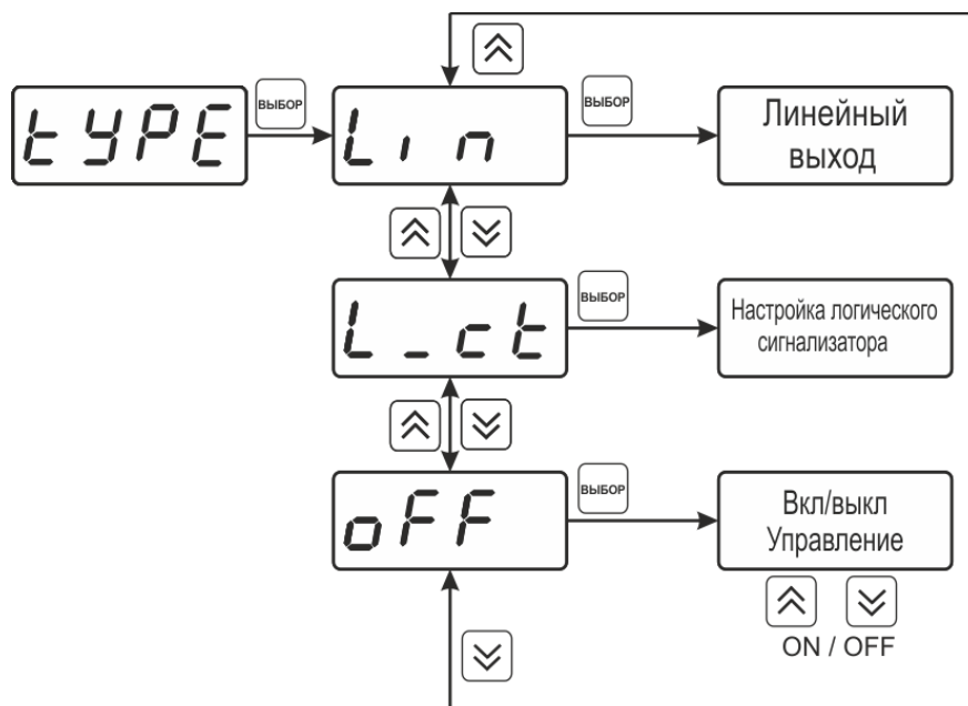
Рисунок 6.27 Выбор логики работы канала управления (токовый выход)
