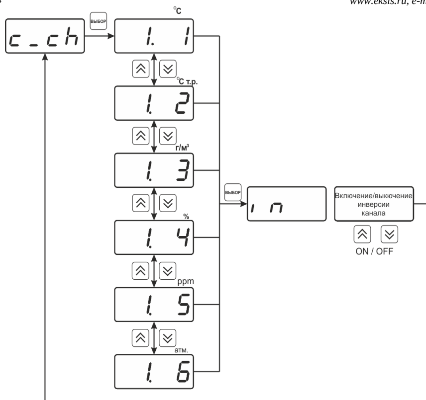
Рисунок 6.24 Настройка входного параметра канала управления (реле)
