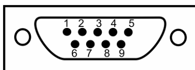
Рисунок 3.6 Разъем подключения прибора к компьютеру по RS-232
