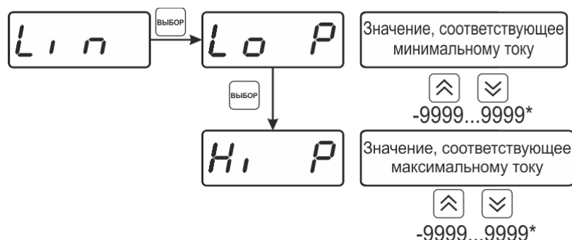
Рисунок 6.30 Настройка линейного выхода
