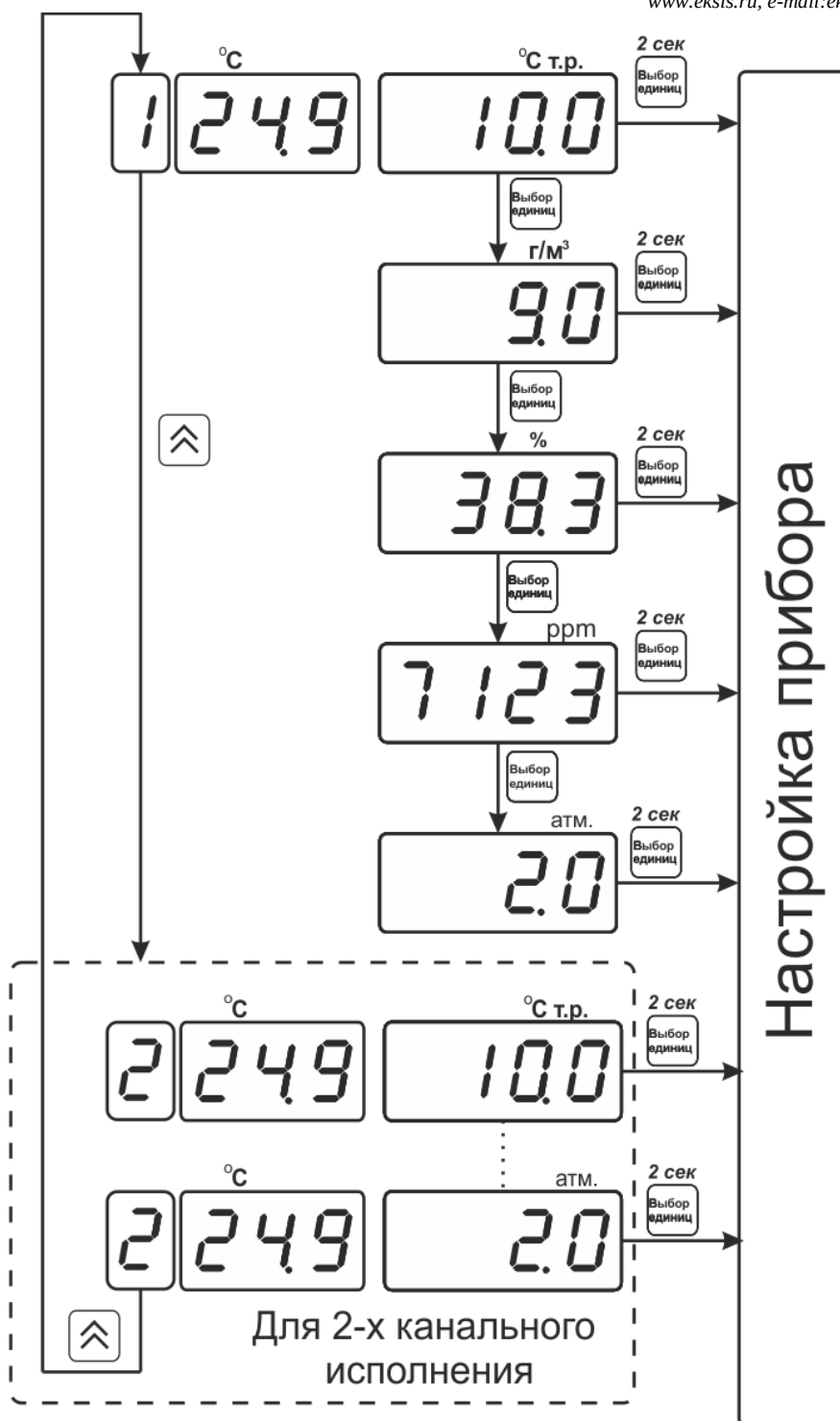
Рисунок 6.2 Режим РАБОТА для двухканального исполнения
